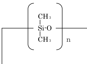
図4 シクロシロキサンの構造式
